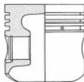
1,5-l-Motor
